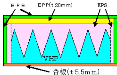
図1 ECCOSORB® VHP-FLの構造
