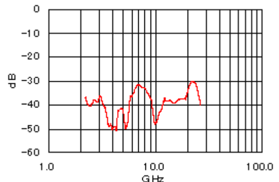
図2 反射減衰量 (VHP-18FL : 代表値)
